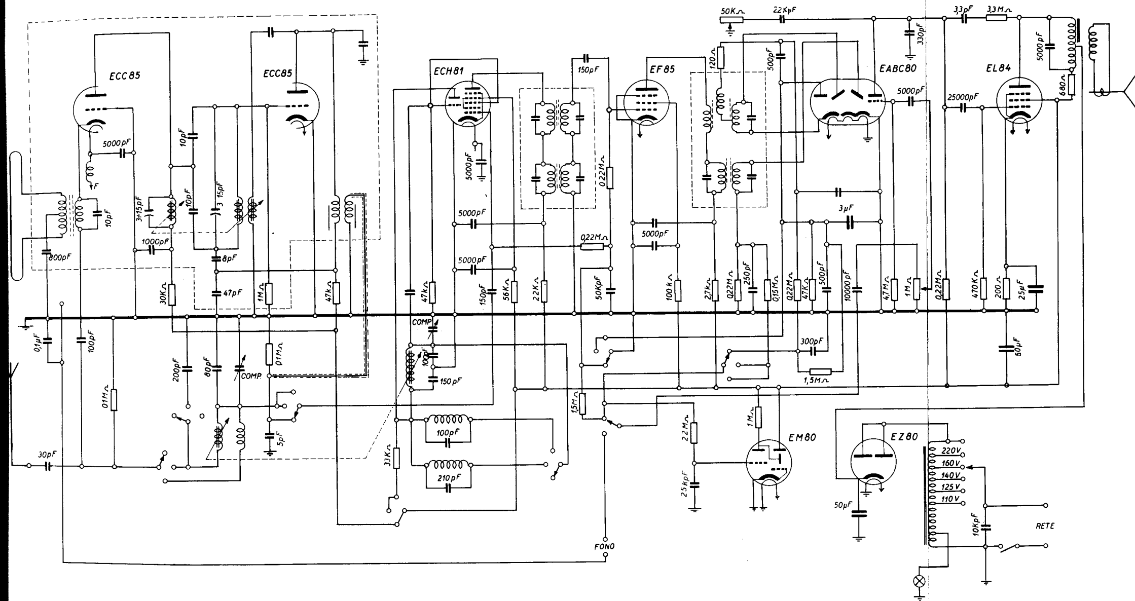
RADIO ALLOCCHIO BACCHINI - Mod. 551. Apparecchio AM/FM, con una gamma onde medie (AM) e una gamma onde ultracorte (FM). Sintonia a permeabilità variabile. Medie frequenze a 465 kc/s e a 10,7 Mc/s. Potenza d'uscita 2,5 watt indistorti. Consumo 45 watt.
